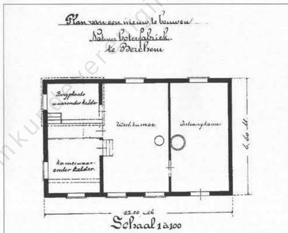
Plattegrond handkracht boterfabriek aan de Laanderstraat.
