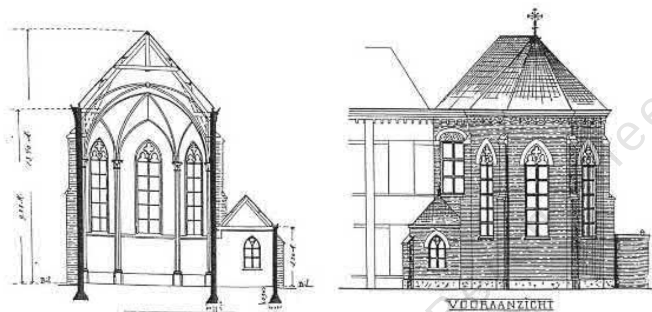
Vooraanzicht kapel + doorsnede.
